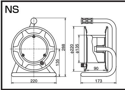
■空リール寸法表 (単位: mm)
