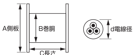
各種コードリール巻取能力表
