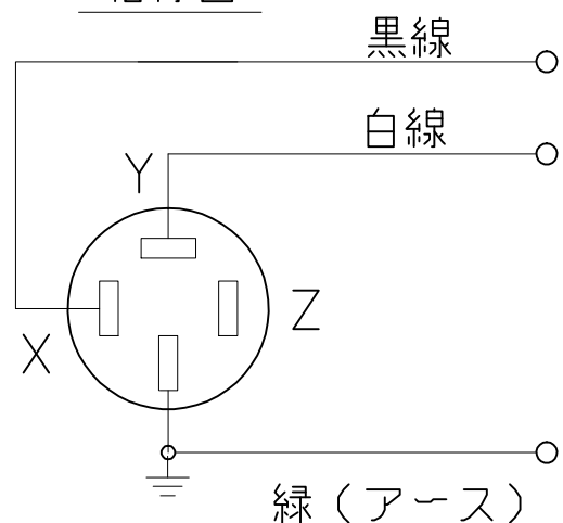
結線図
