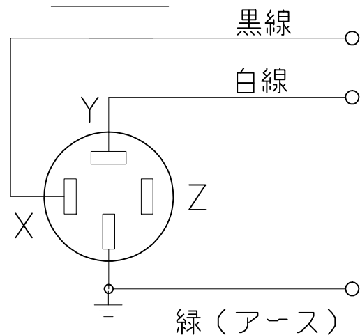
結線図
