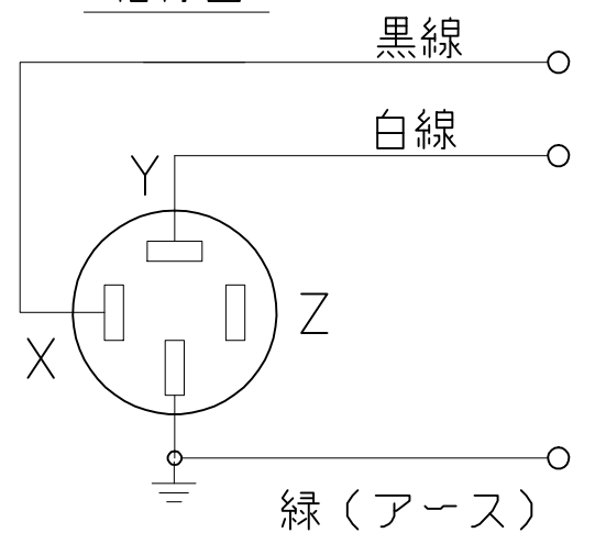
結線図
