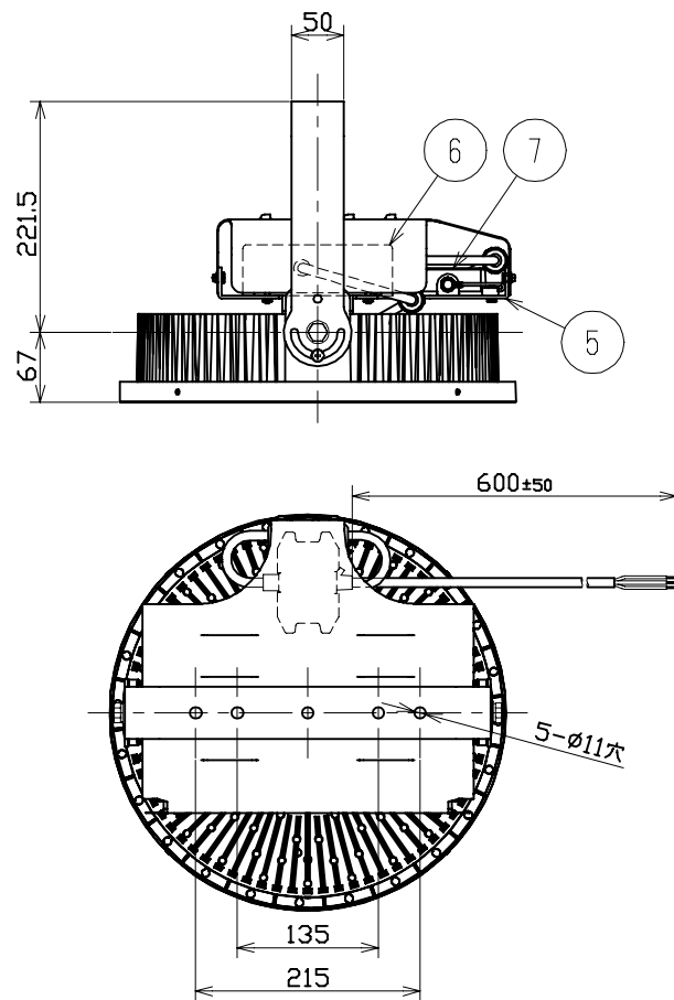
A矢視図
