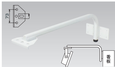
SE-N10T2 (アーム エルボーTYPE2)
