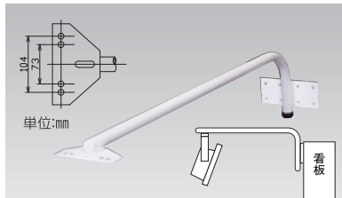
SE-T2 (アーム エルボーTYPE2)
