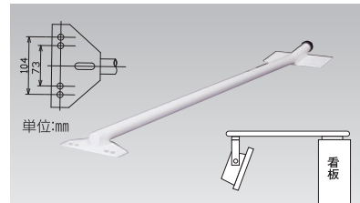
SS-900 (アーム ストレート)
