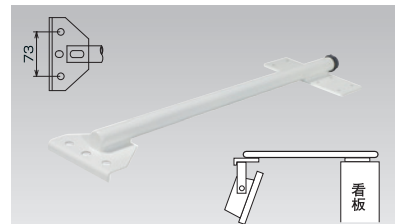
SS-N10 (アーム ストレート)
