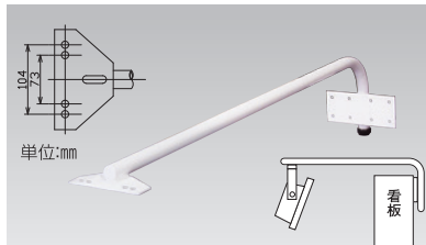
SE-T1 (アーム エルボーTYPE1)
